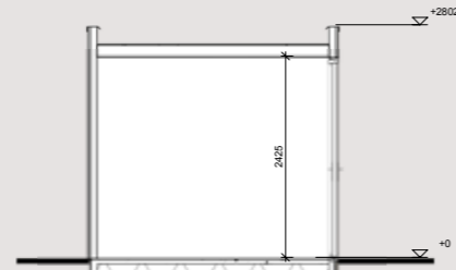
doorsnede
