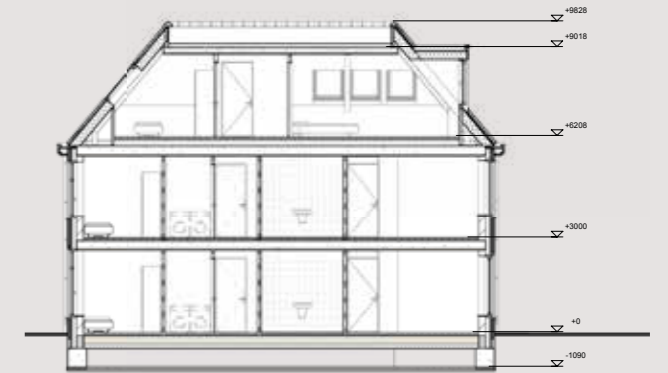
Doorsnede
