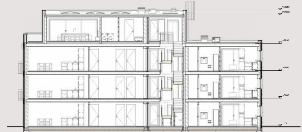
Doorsnede
